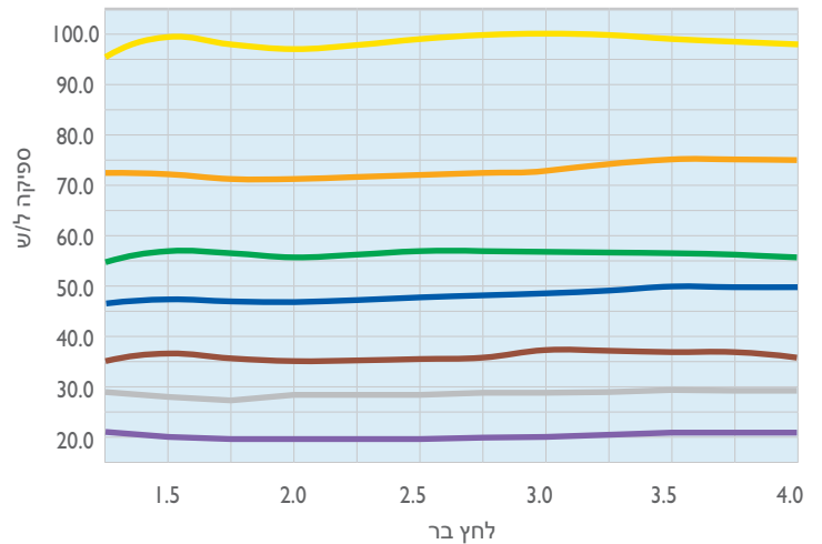
תלות ספיקה בלחץ
